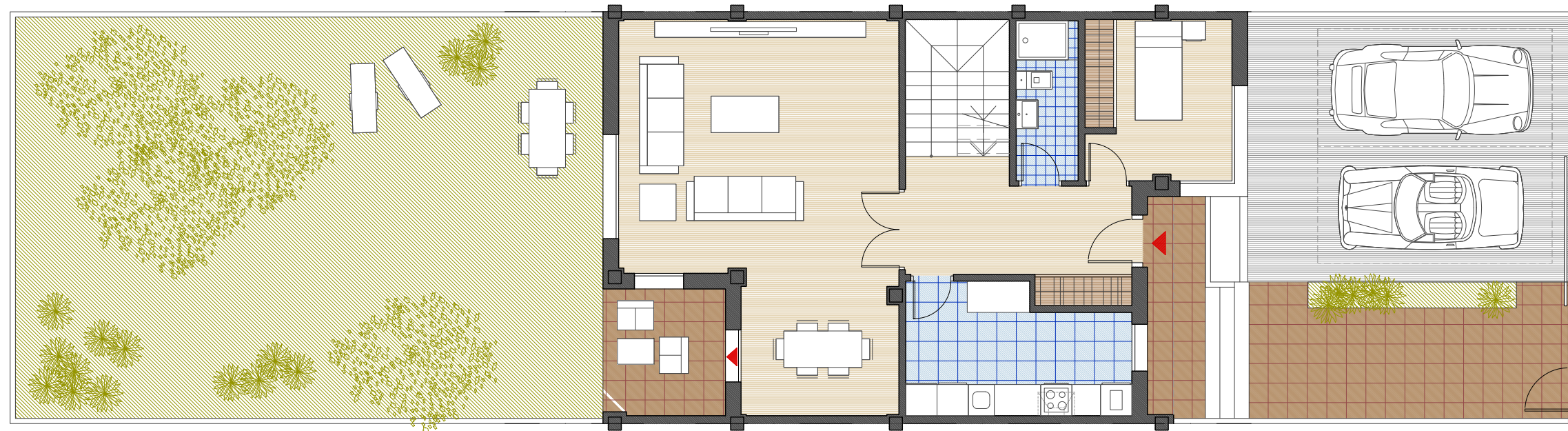
PLANTA BAJA
